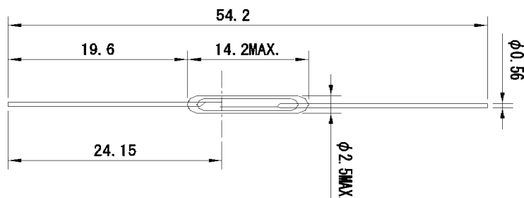
寸法 Dimensions
