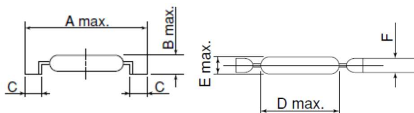
寸法 Dimensions
