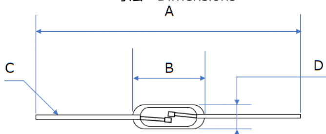
寸法 Dimensions
